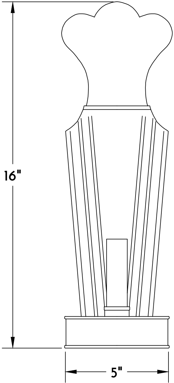
① SCONCE FRONT ELE.
