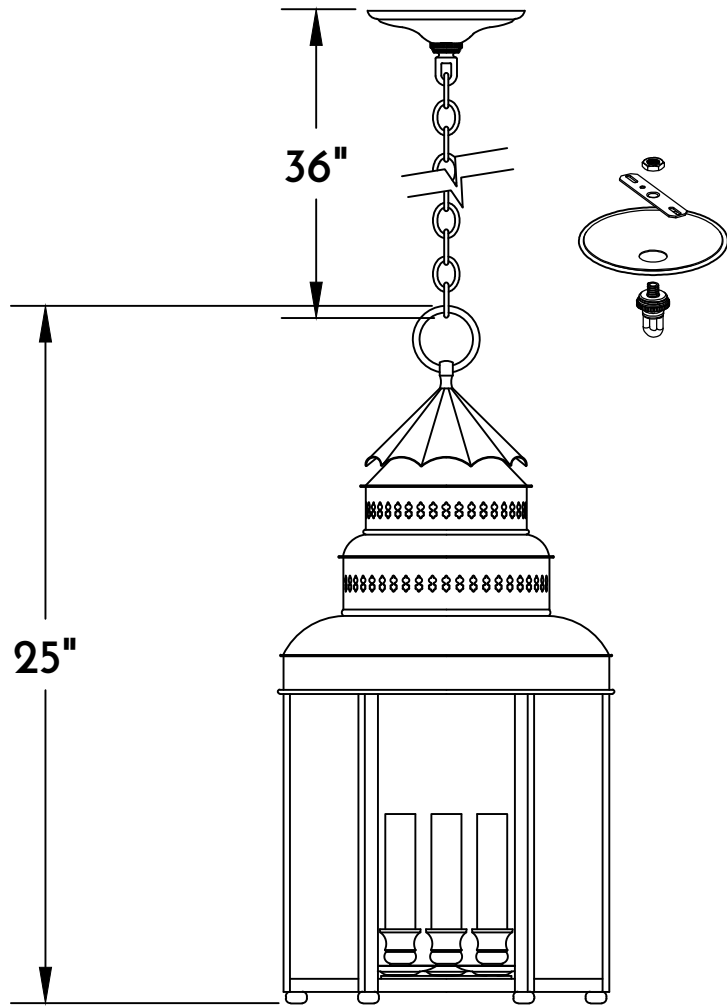
① LANTERN SIDE ELE.
