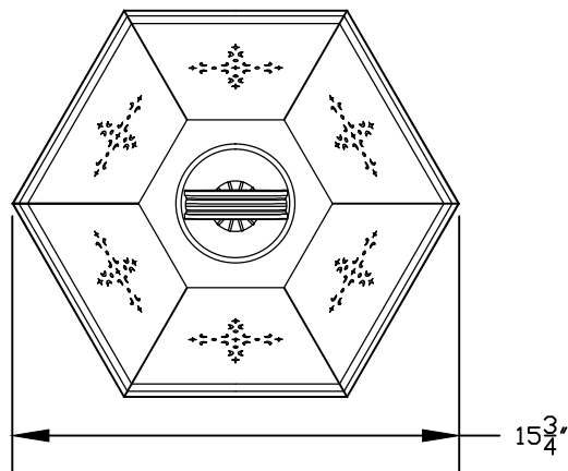
3 WALL PENDANT PLAN VIEW
